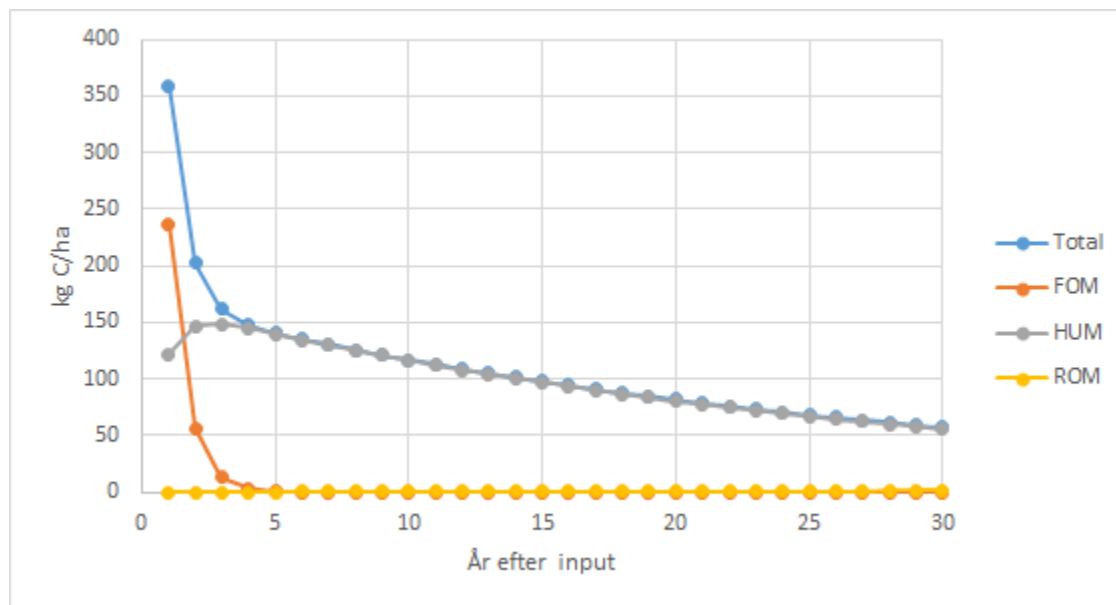
Figur 4.3.1 Ændringer i kulstoflagring i frisk organisk stof (FOM), humus organisk stof (HUM), resistent organisk stof (ROM) og total-kulstof over tid, efter 1 \text{ t ha}^{-1} kulstofinput som FOM. Nedbrydningsrater; frisk organisk stof (FOM) = 1,44 \text{ år}^{-1} , humus organisk stof (HUM) = 0,0366 \text{ år}^{-1} , resistent organisk stof (ROM) = 4,63 \times 10^{-4} \text{ år}^{-1} , humification = 0,16, romification = 0,012.
