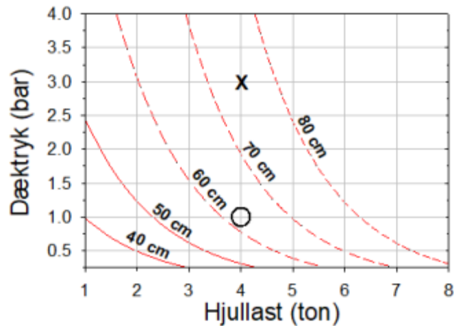
Figur 4.1 - Den forventede, mekaniske styrke i vintervåd jord i dybden, hvor der trykkes med 0,5 bar ved forskellige dæktryk og hjullast. Eksempel: En hjullast på 4 ton og et dæktryk på 3 bar, vil pakke jorden til ca. 75 cm dybde, når der køres på vintervåd jord (figurens X). Ved at reducere dæktrykket til 1 bar reduceres pakkedybden med næsten 15 cm (figurens O). (Askegaard et al., 2021).
